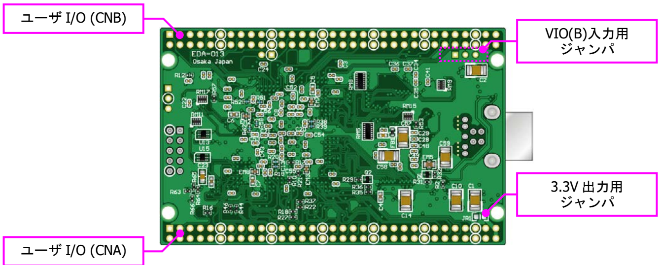
はんだ面
