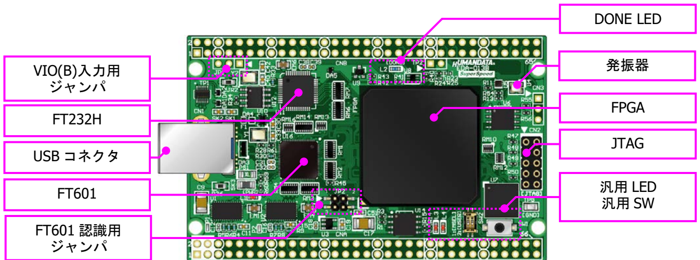
部品面
