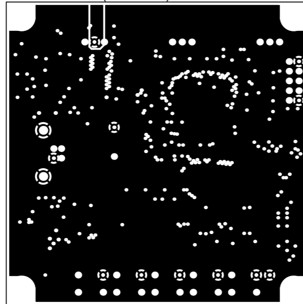
InternalPlane1 (Scale 1:1)
