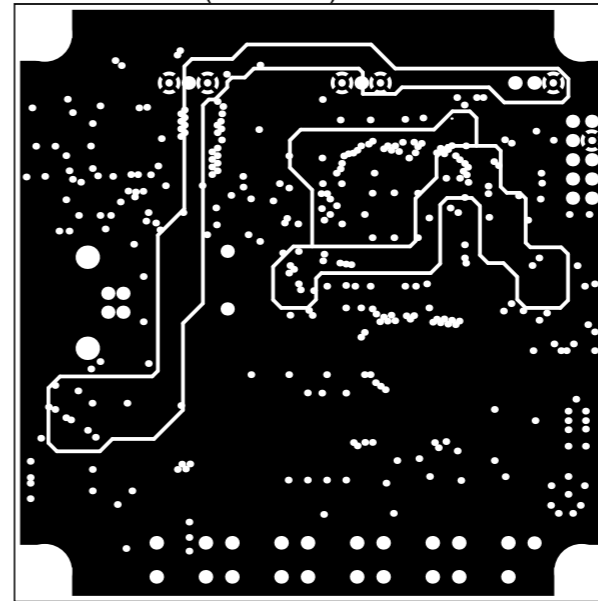
InternalPlane2 (Scale 1:1)
