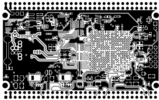
TOP LAYER
