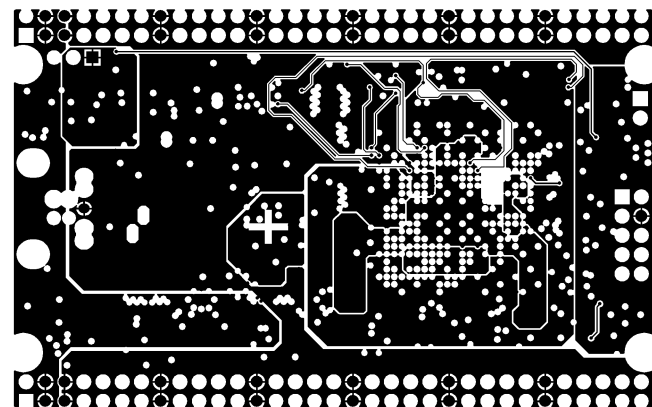
MID LAYER1
