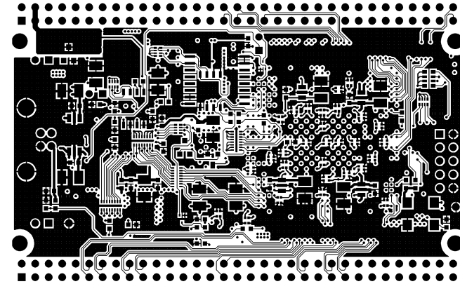
BOTTOM LAYER
