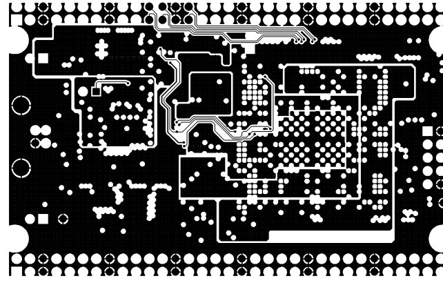
MID LAYER2
