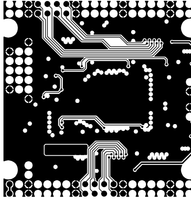
MID LAYER2
