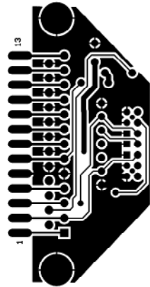
TOP LAYER
