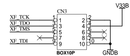
JTAGコネクタ
