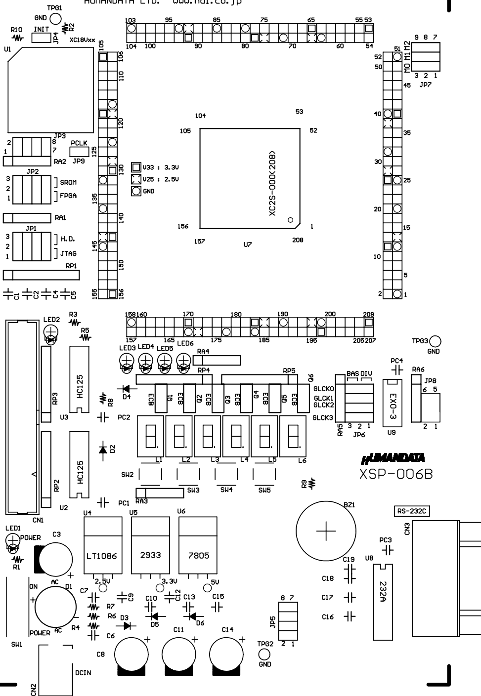
Top Overlay
