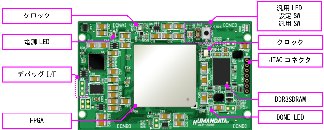
部品面
