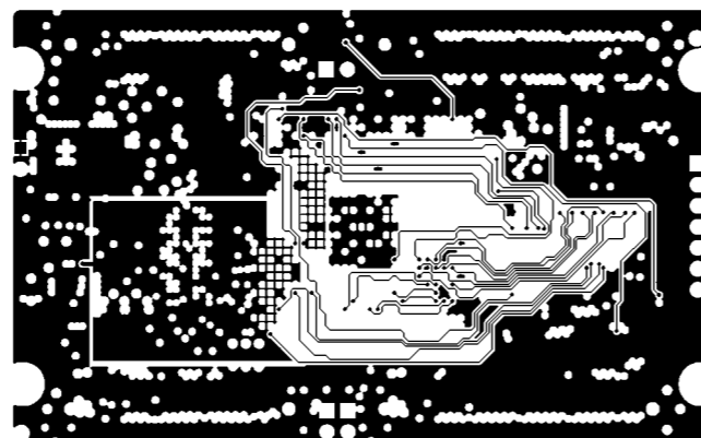
MID LAYER 5
