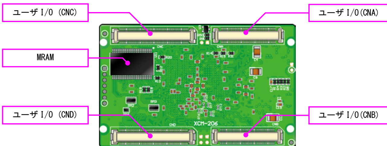
はんだ面
