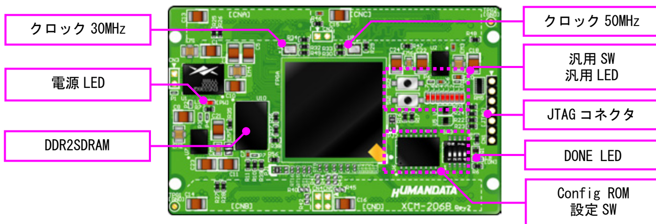
部品面
