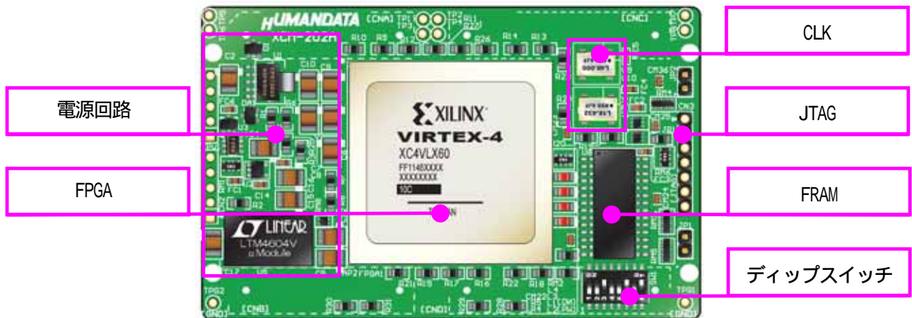
部品面
