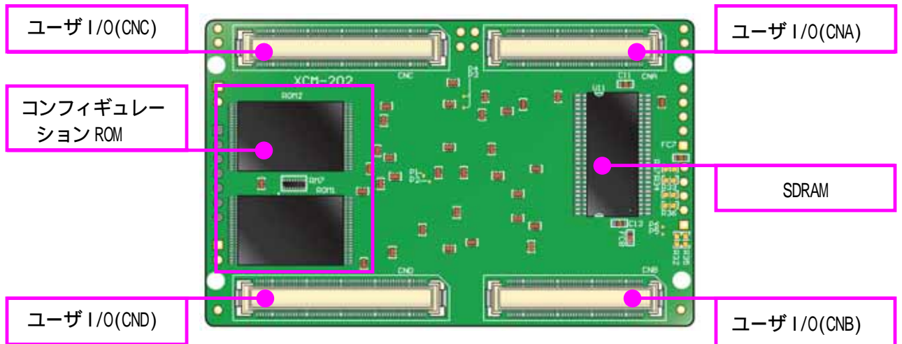
はんだ面
