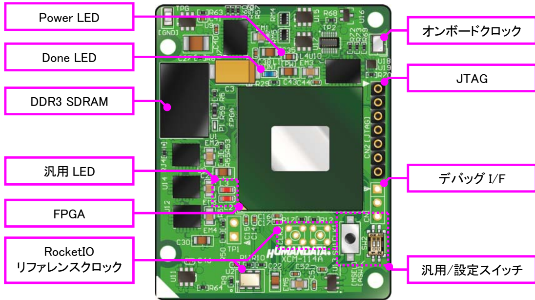
部品面
