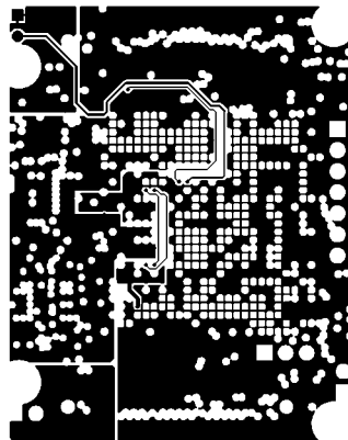
MID LAYER2
