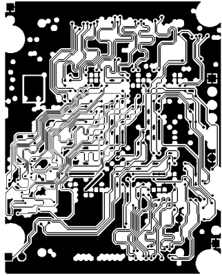
MID LAYER1
