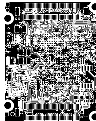
BOTTOM LAYER
