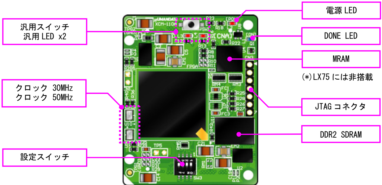
部品面
