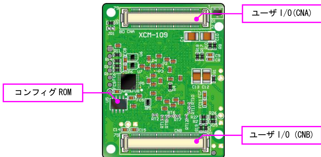
はんだ面
