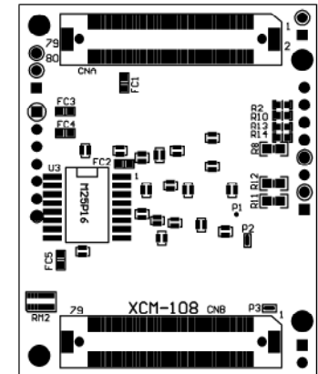
はんだ面
