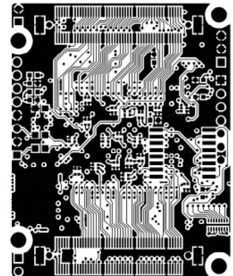
BOTTOM LAYER
