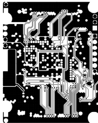
MID LAYER1
