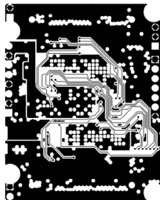
MID LAYER2
