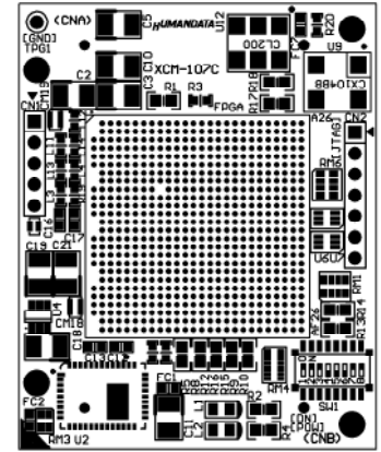
部品面
