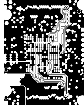
MID LAYER 3
