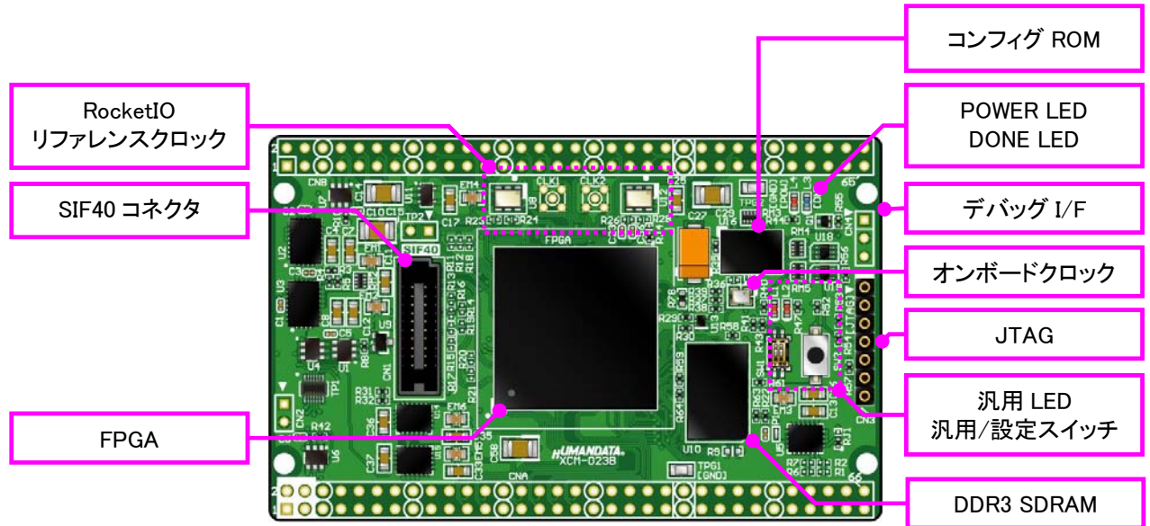
部品面
