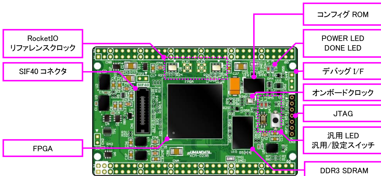
部品面
