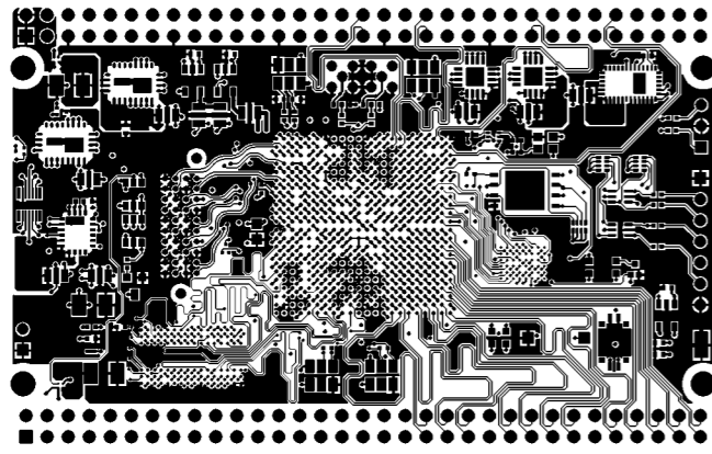
TOP LAYER
