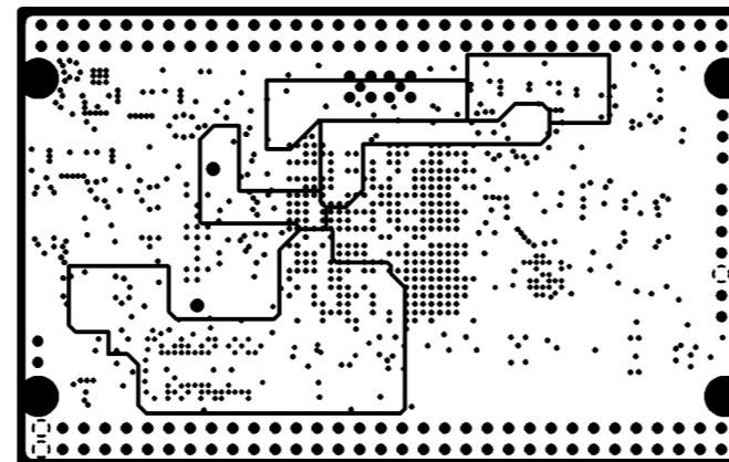
MID LAYER2
