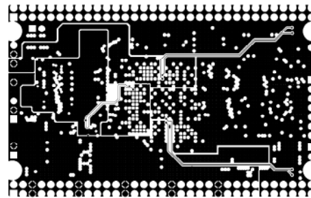
MID LAYER2
