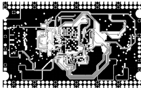
MID LAYER1
