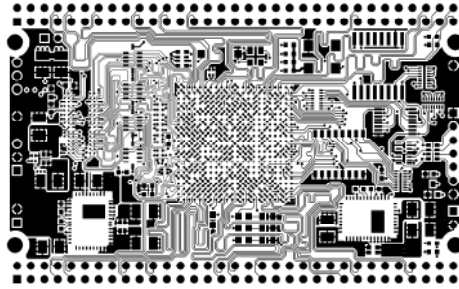
TOP LAYER
