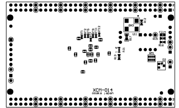
はんだ面
