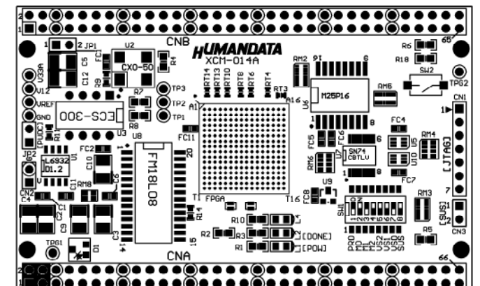
部品面
