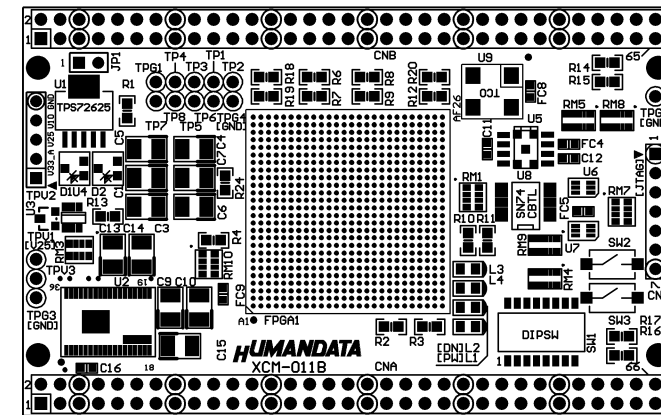
部品面
