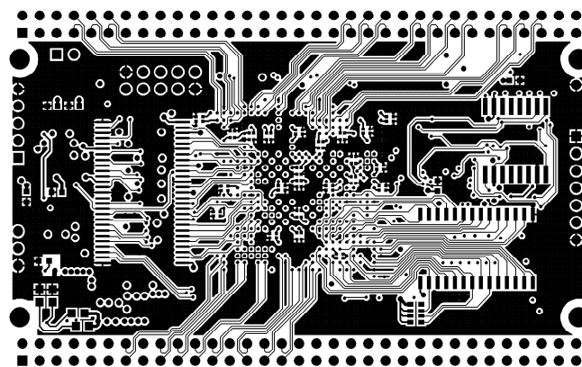
BOTTOM LAYER
