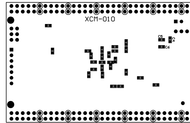
はんだ面
