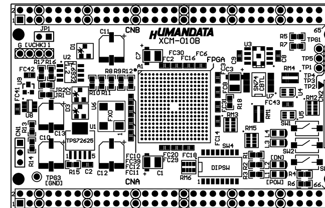
部品面
