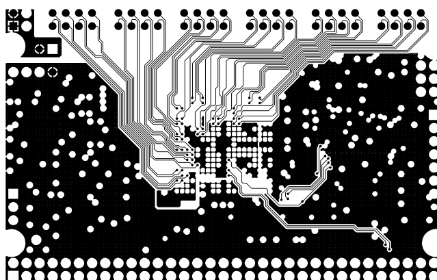
MID LAYER 2
