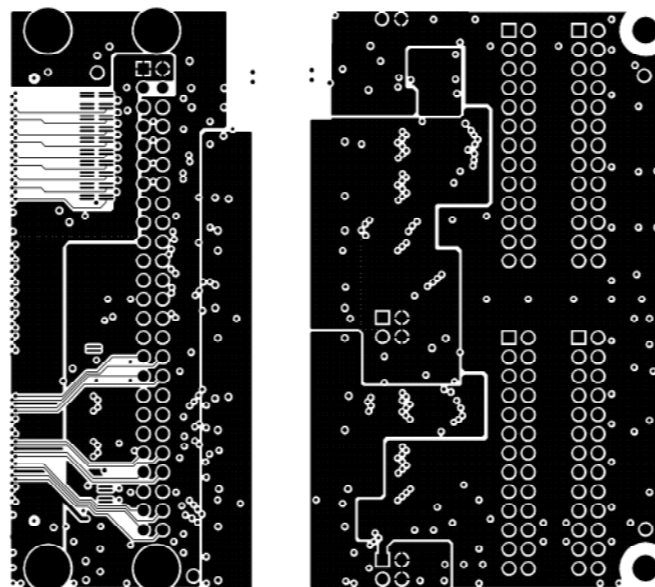
MID LAYER
