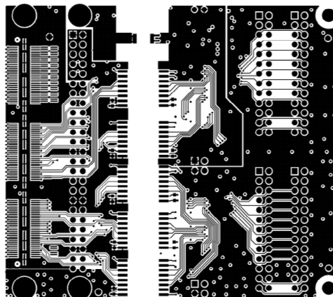
BOTTOM LAYER
