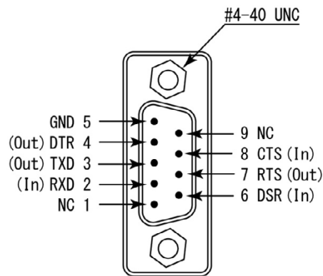
D-Sub9 ピン (オス)
