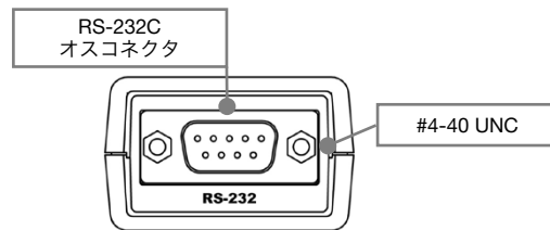
RS-232 側パネル
