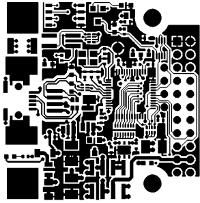
TOP LAYER
