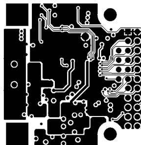
BOTTOM LAYER
