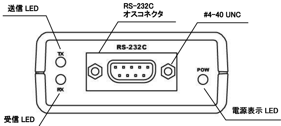
RS-232 側パネル
