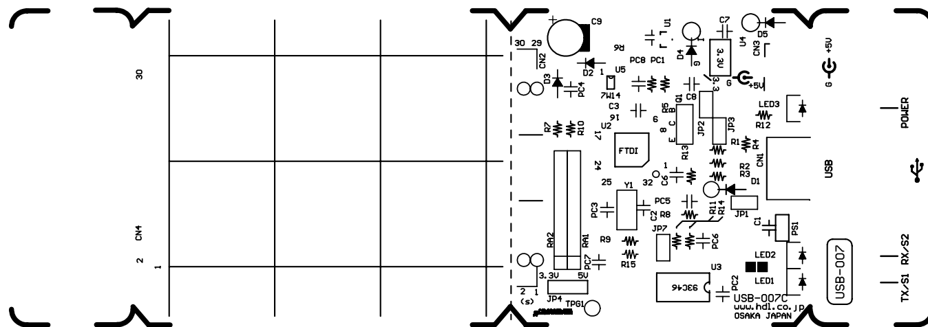
Top Overlay
