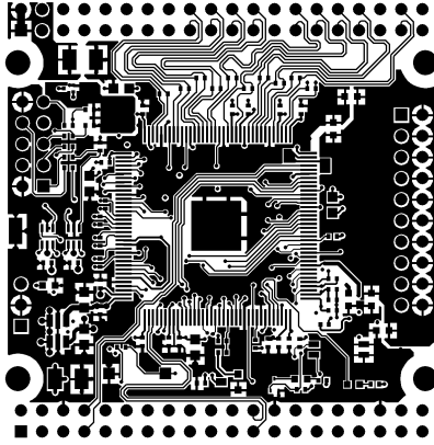
TOP LAYER
