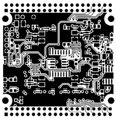
BOTTOM LAYER
