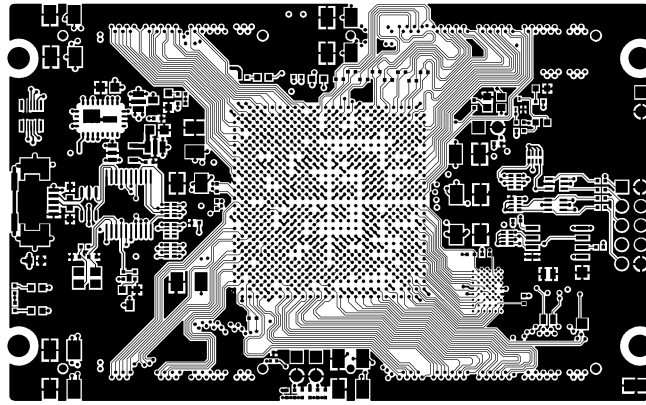
TOP LAYER
