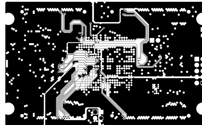
MID LAYER 2
