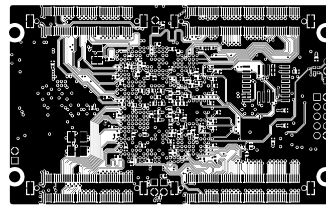
BOTTOM LAYER
