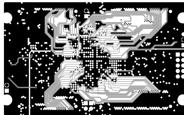
MID LAYER 2
