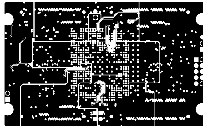
MID LAYER 3
