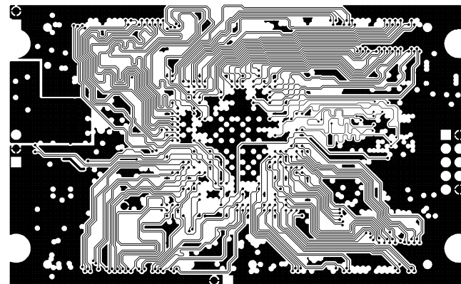
MID LAYER 1
