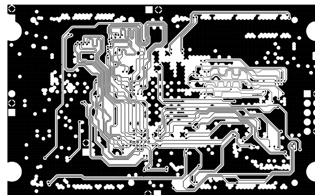
MID LAYER 2
