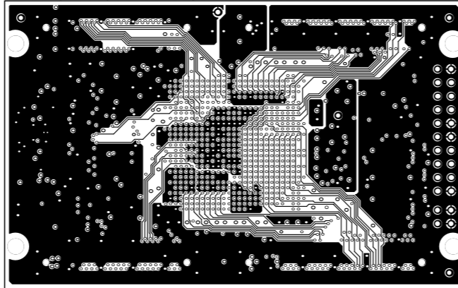
InternalPlane1 (Scale 1:1)
