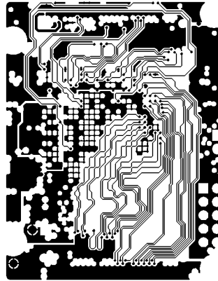
MID LAYER2
