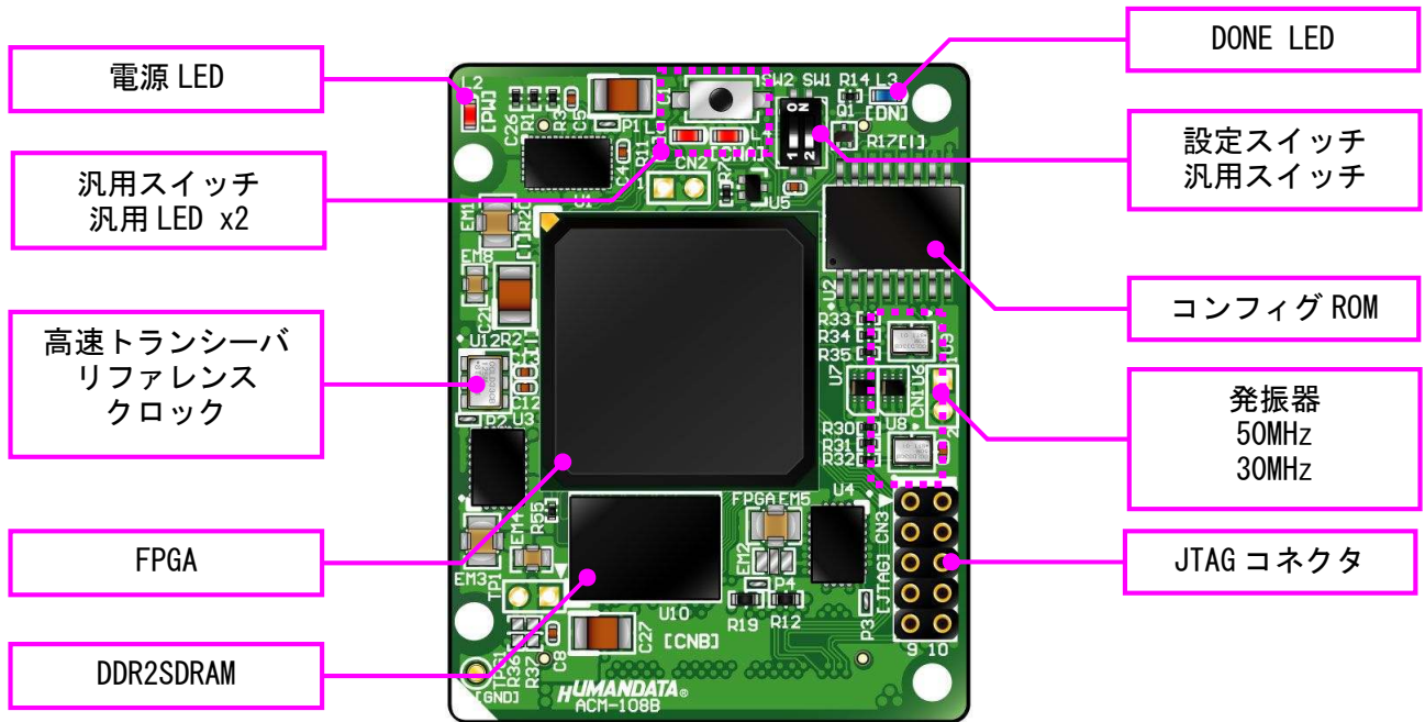
部品面
