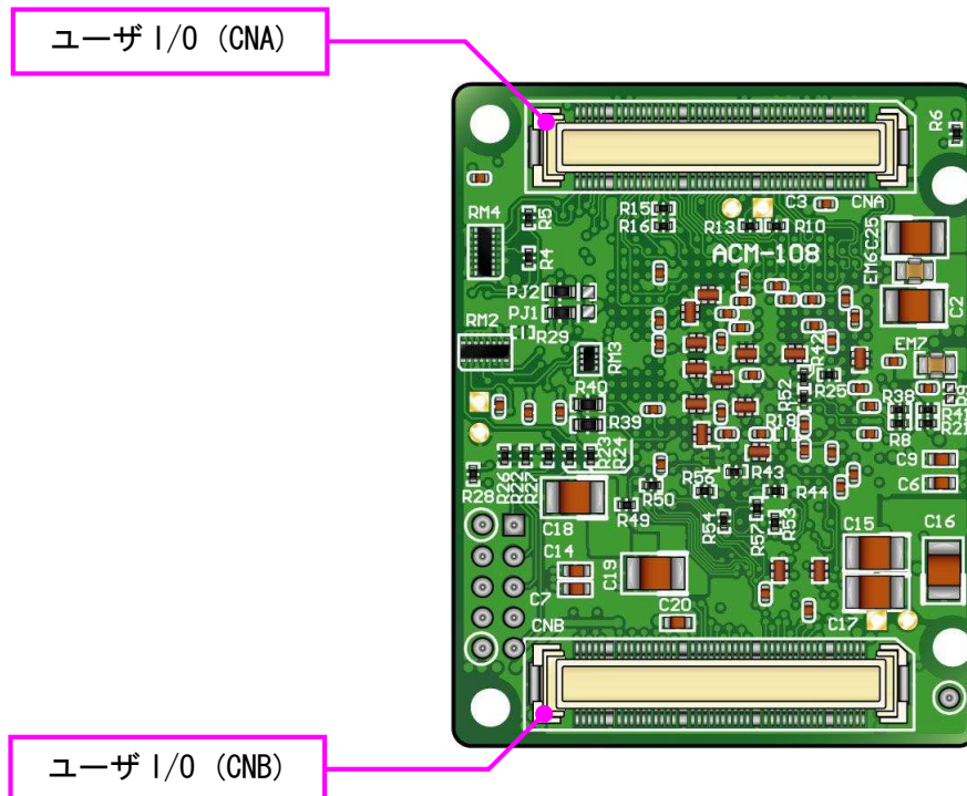
はんだ面
