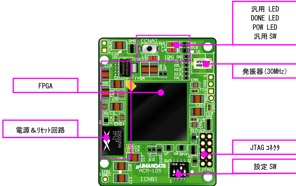
部品面
