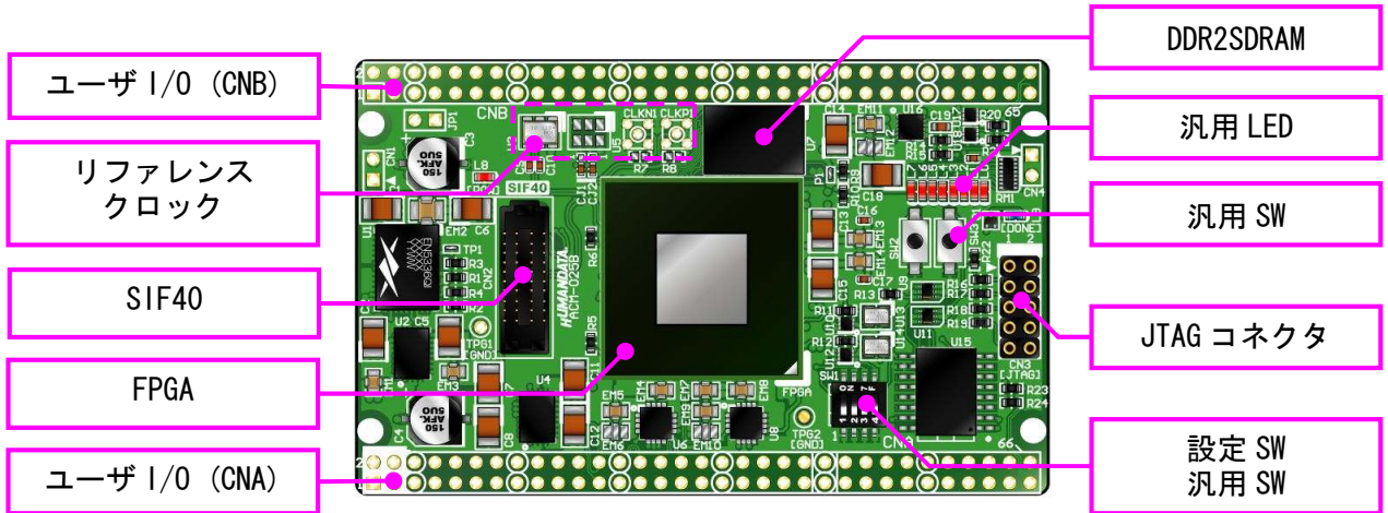
部品面
