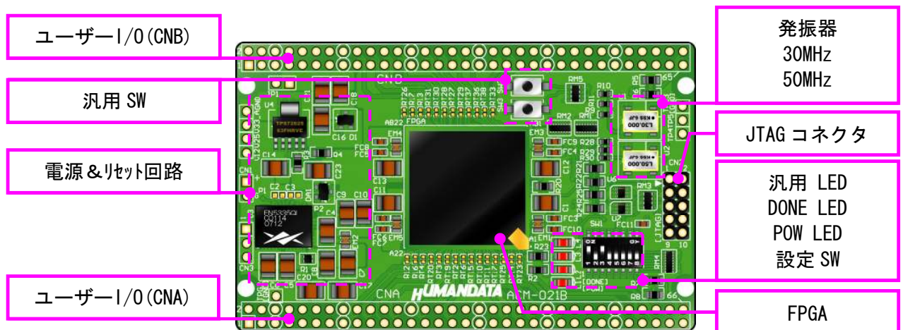
部品面
