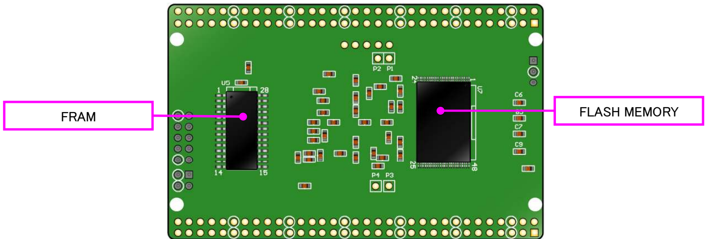
はんだ面
