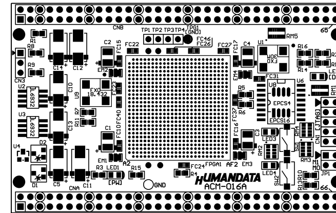
部品面
