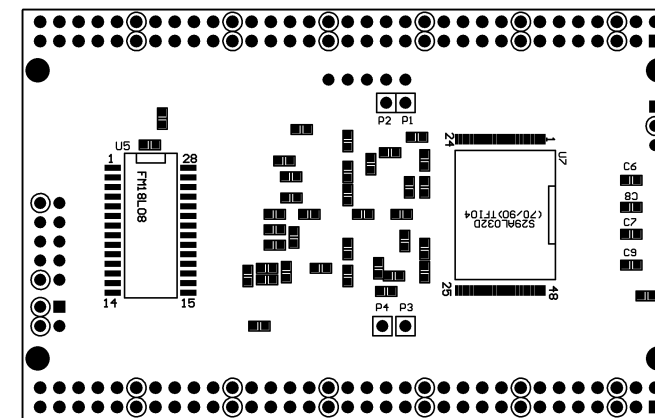
はんだ面
