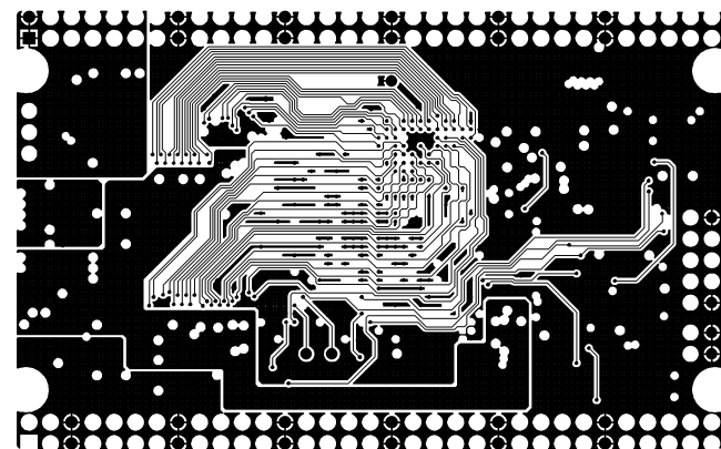
MID LAYER 1
