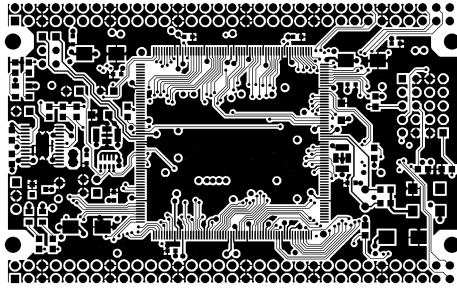
TOP LAYER
