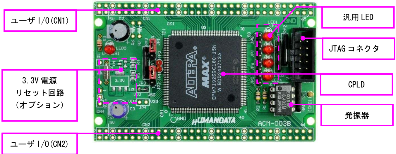
部品面
