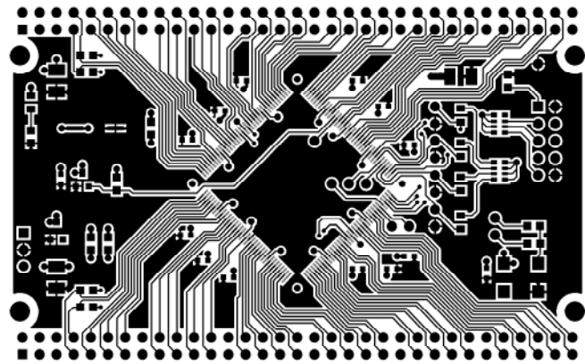
TOP LAYER
