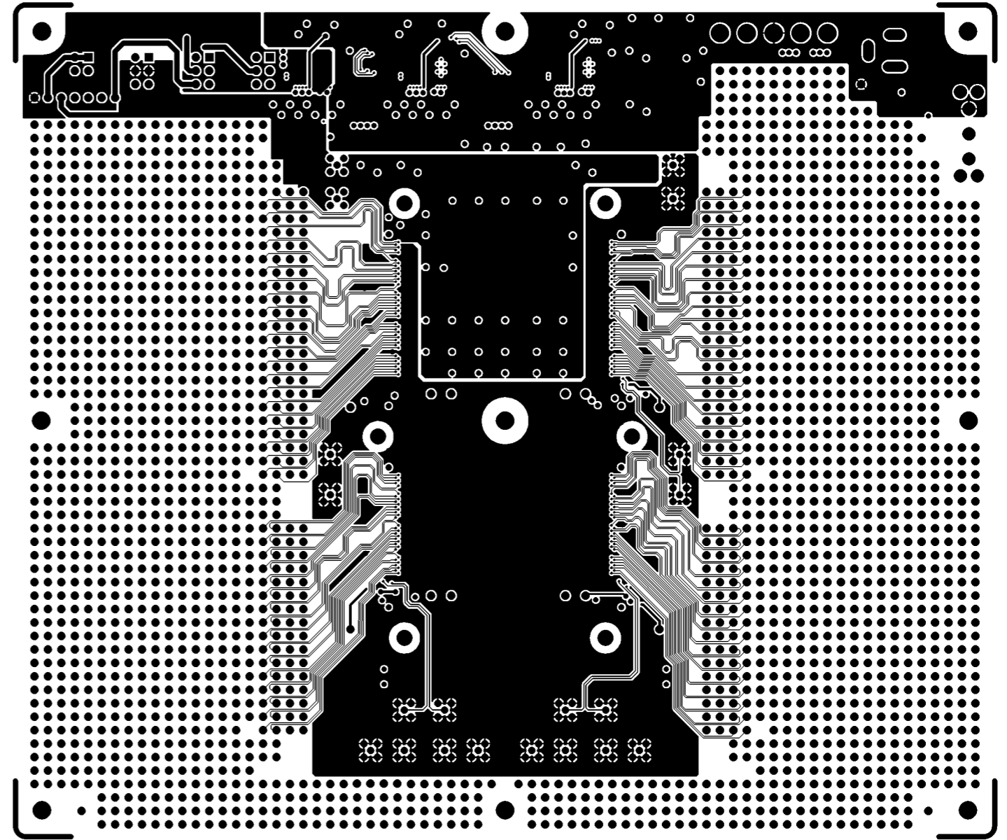
BOTTOM LAYER
