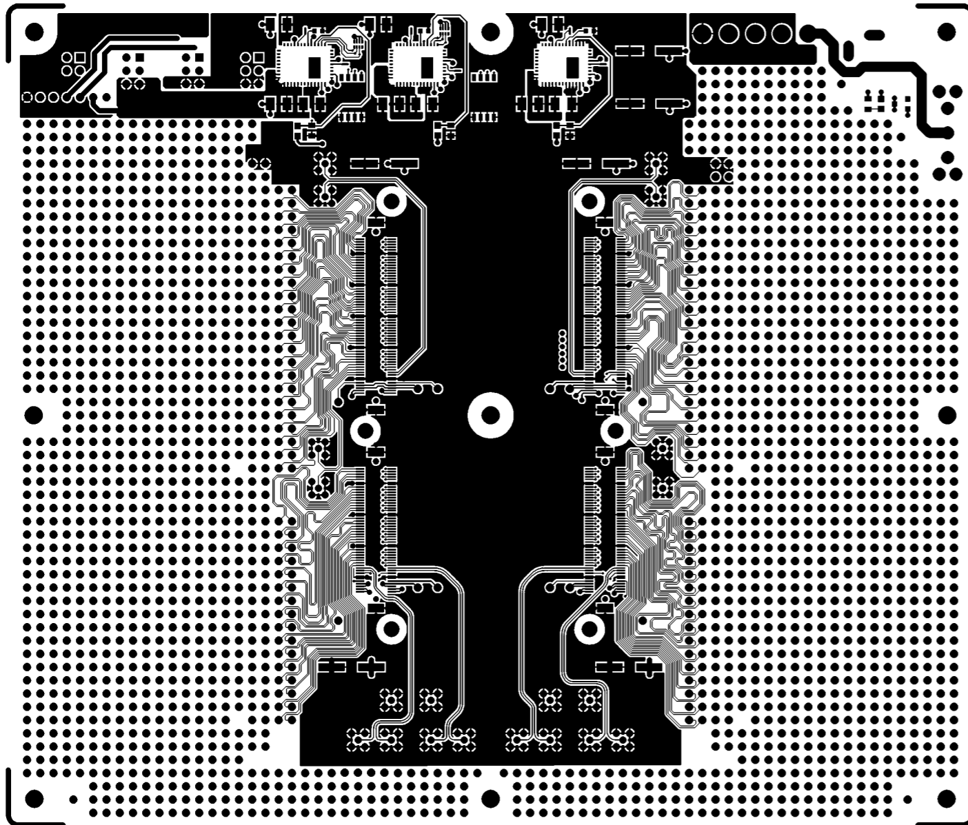
TOP LAYER
