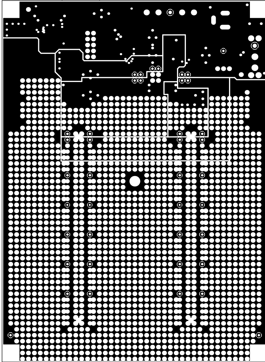
InternalPlane2 (Scale 1:1)
