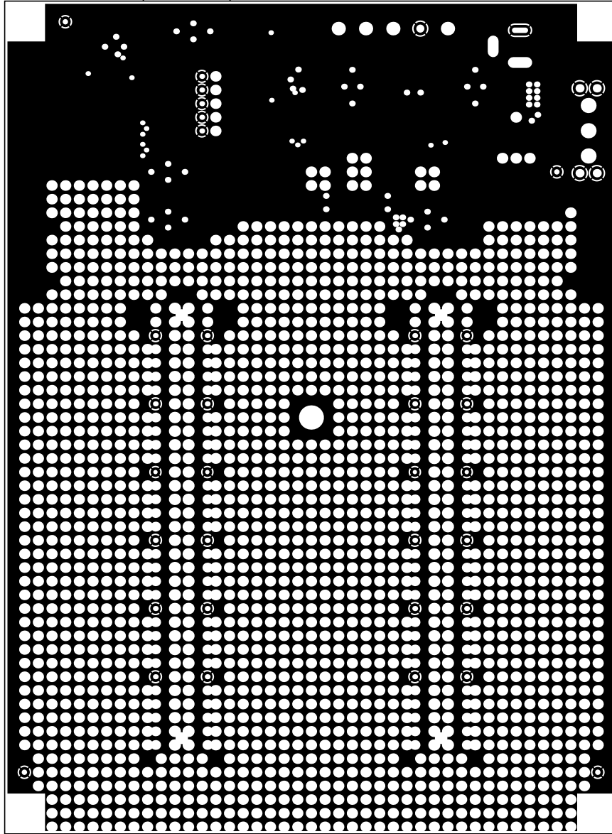
InternalPlane1 (Scale 1:1)
